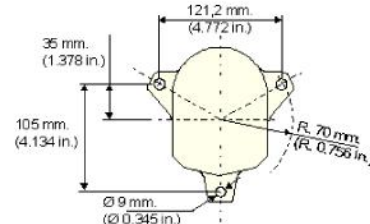
УСТАНОВКА НА ОПОРНОЙ ПЛИТЕ
